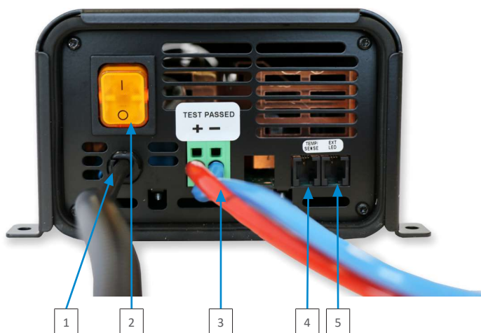
Abb. 2: Ladegerät ABC Anschlussseite
